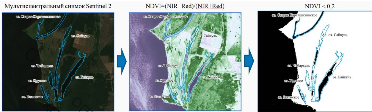
Рис. 2. Использование NDVI для дистанционной оценки зарастания озер
